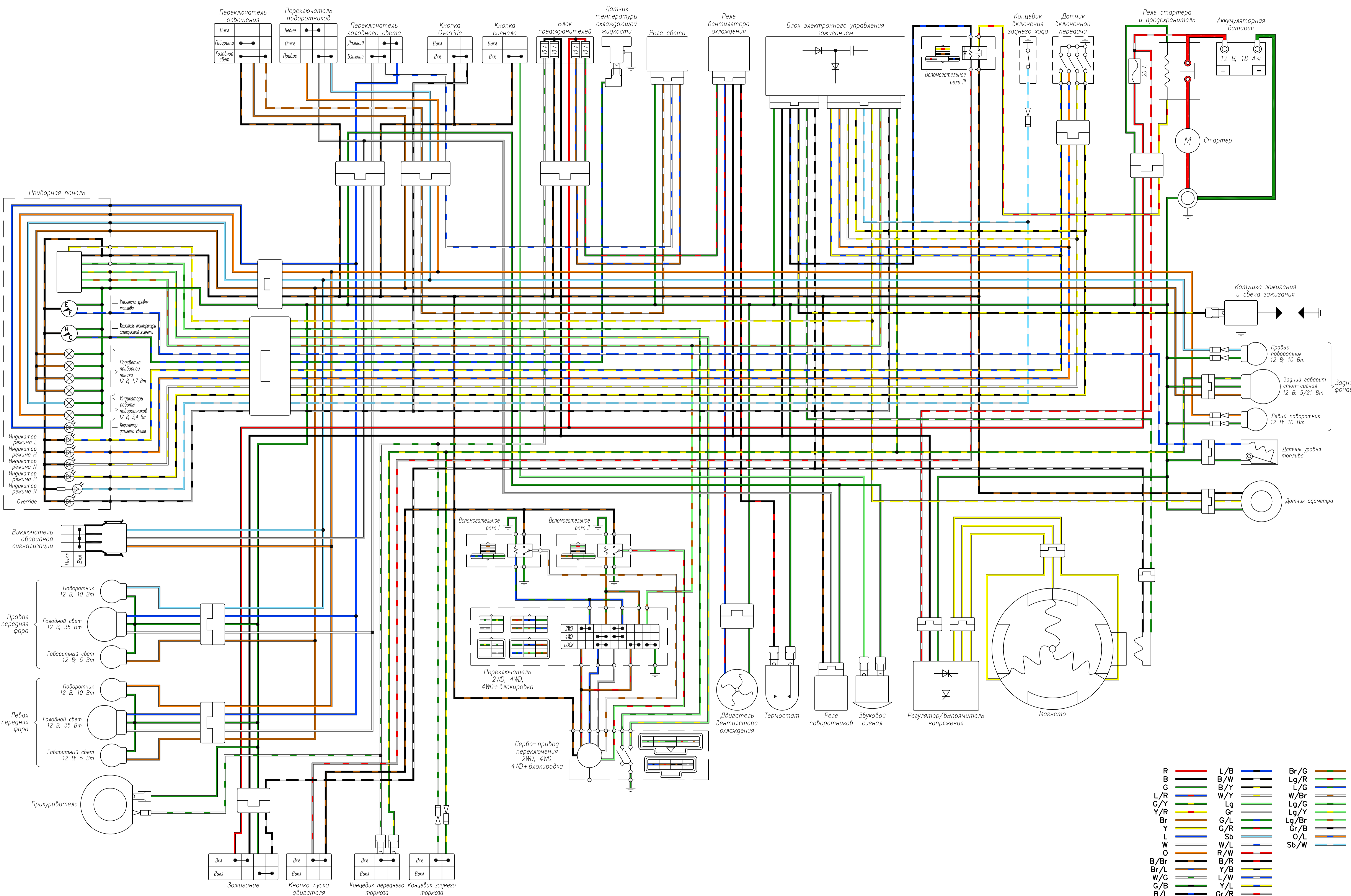
Электрическая схема квадроцикла CFMOTO CF500A
